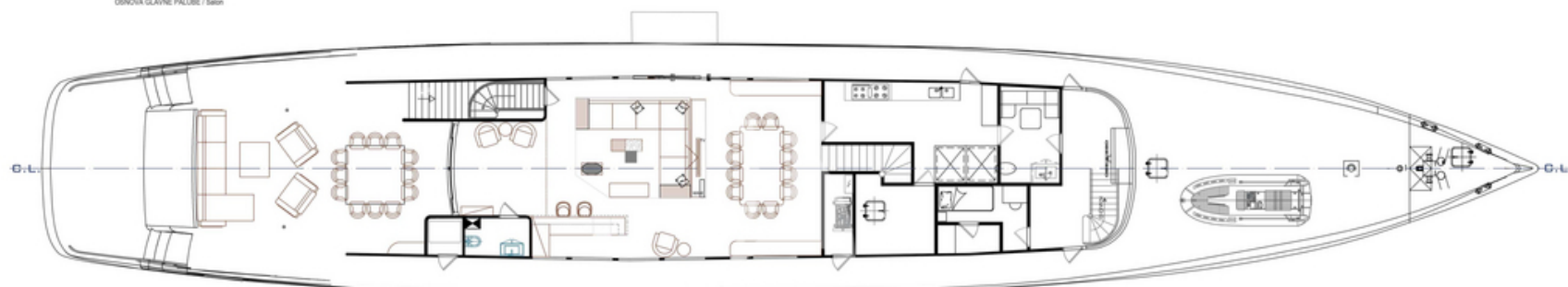
SCORPIOS YACHT OSNOVA GLAVNE PALUBE / Salon
